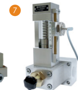
KUI-M Volumetric flow display
